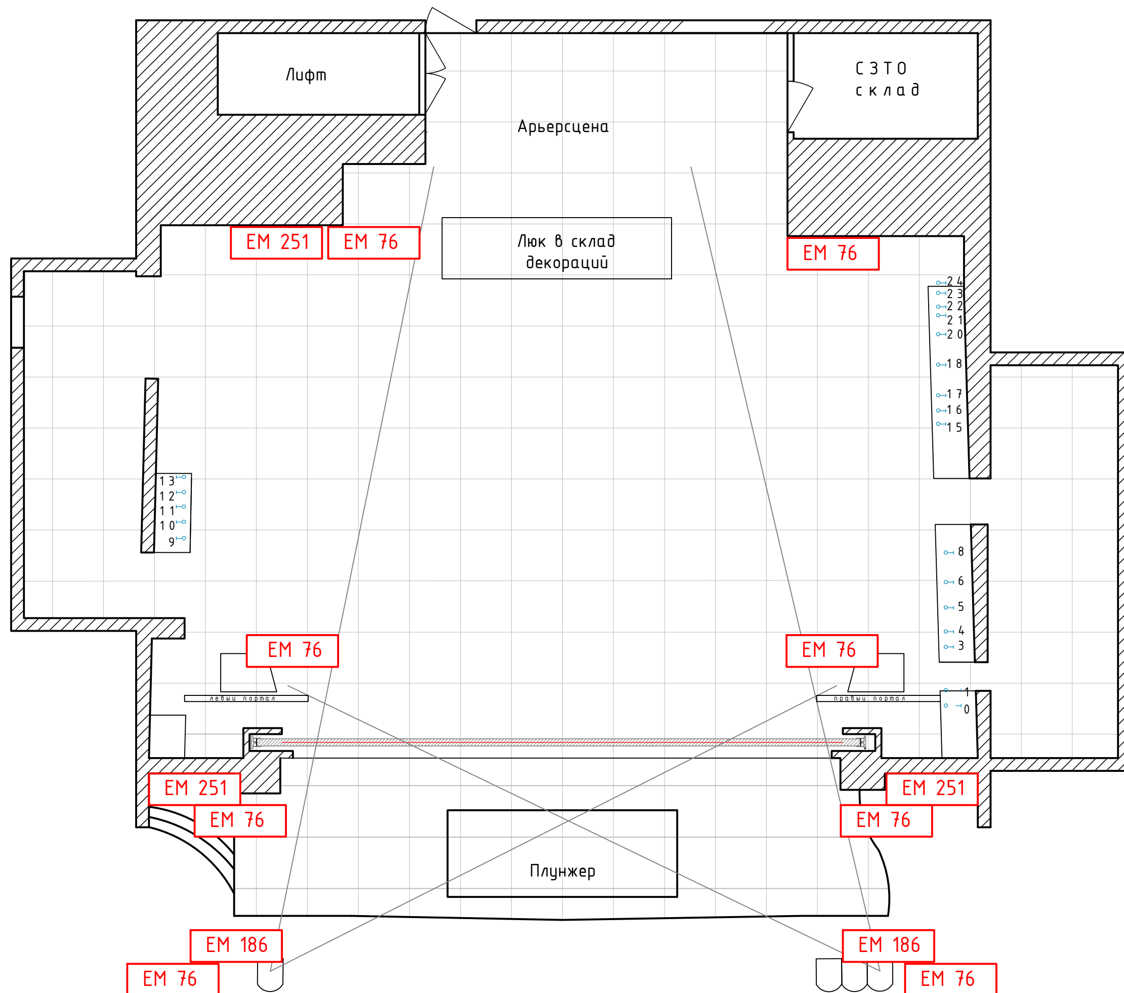
Схема расположения акустических систем.
